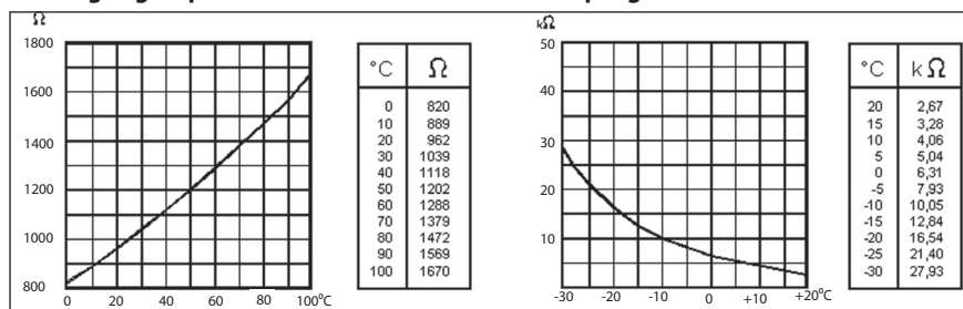
Framledningsgivare T1
