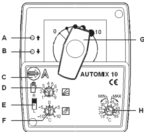
Kuva 2. Säätömoottorin etupinta.
